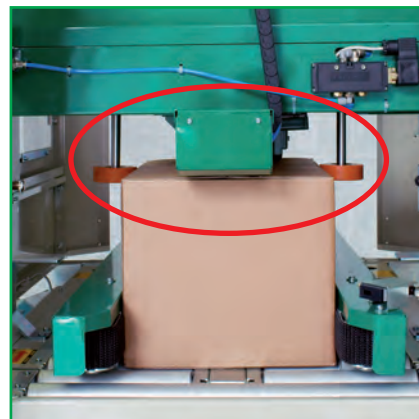
Seitliche obere pneumatische Paket-Andruckrollen für NCX-520, 670, 820.
